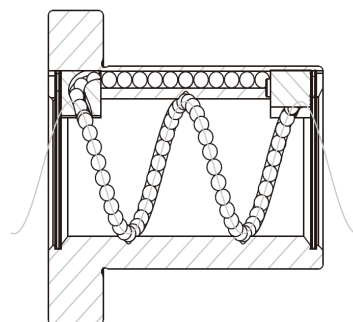
Fig 1.6.5 B - Type Nut
