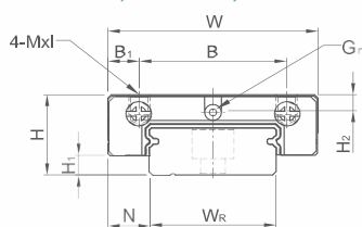
SMW7-0, S MW9-0, S MW12-0
