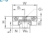
SMN7-0, SMN9-0, SMN12-0
