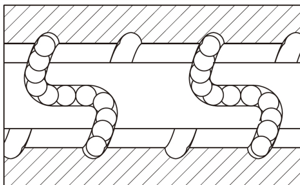
Fig 1.6.2 K - Type Nut
